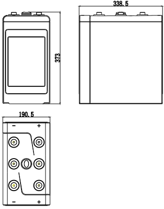
备注：所有尺寸的公差为±2mm：
